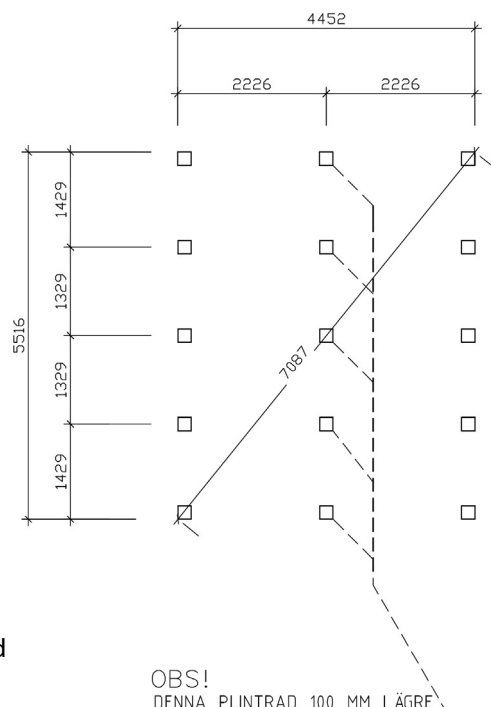
Plintritning
